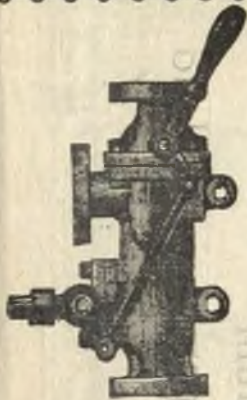
Универс. Инжекторъ
