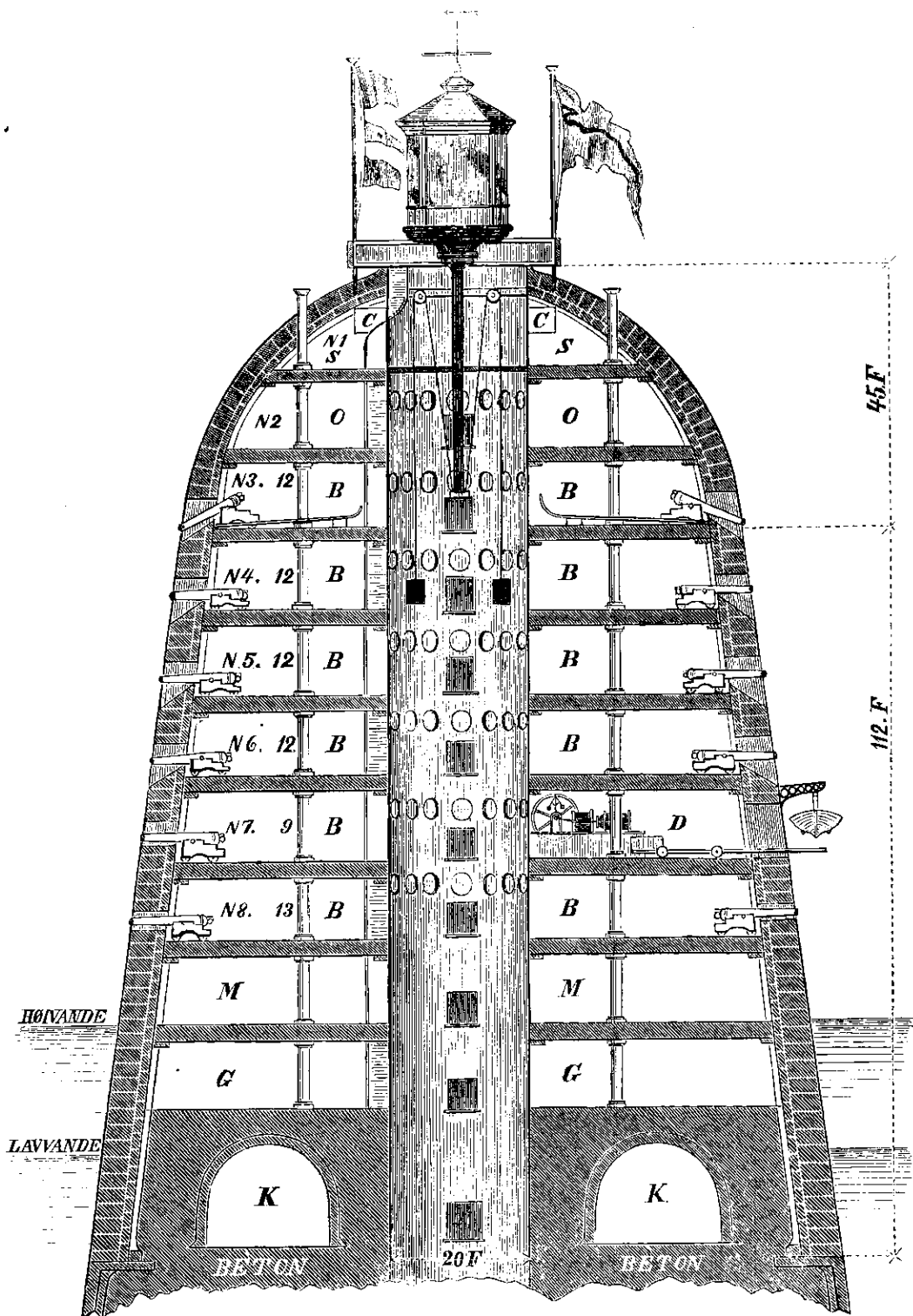
Tværsnit af det vindtagelige Fort.
