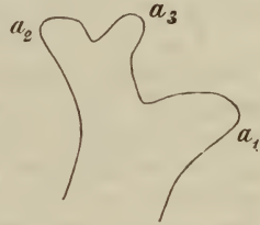
Fig. 14. Sympode dichotome.
