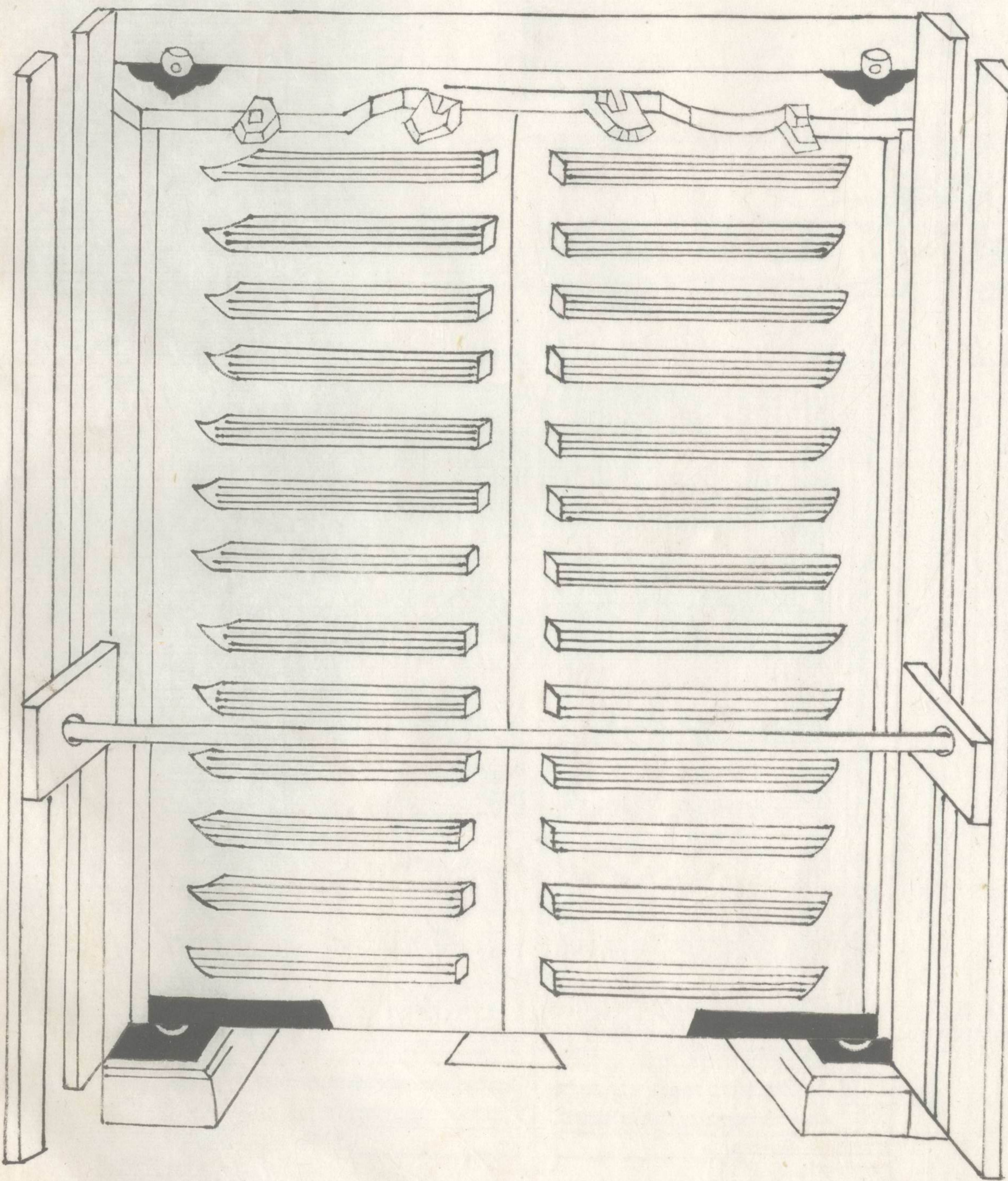
小木作制度圖樣 門憲格子門等第一附 垂魚
