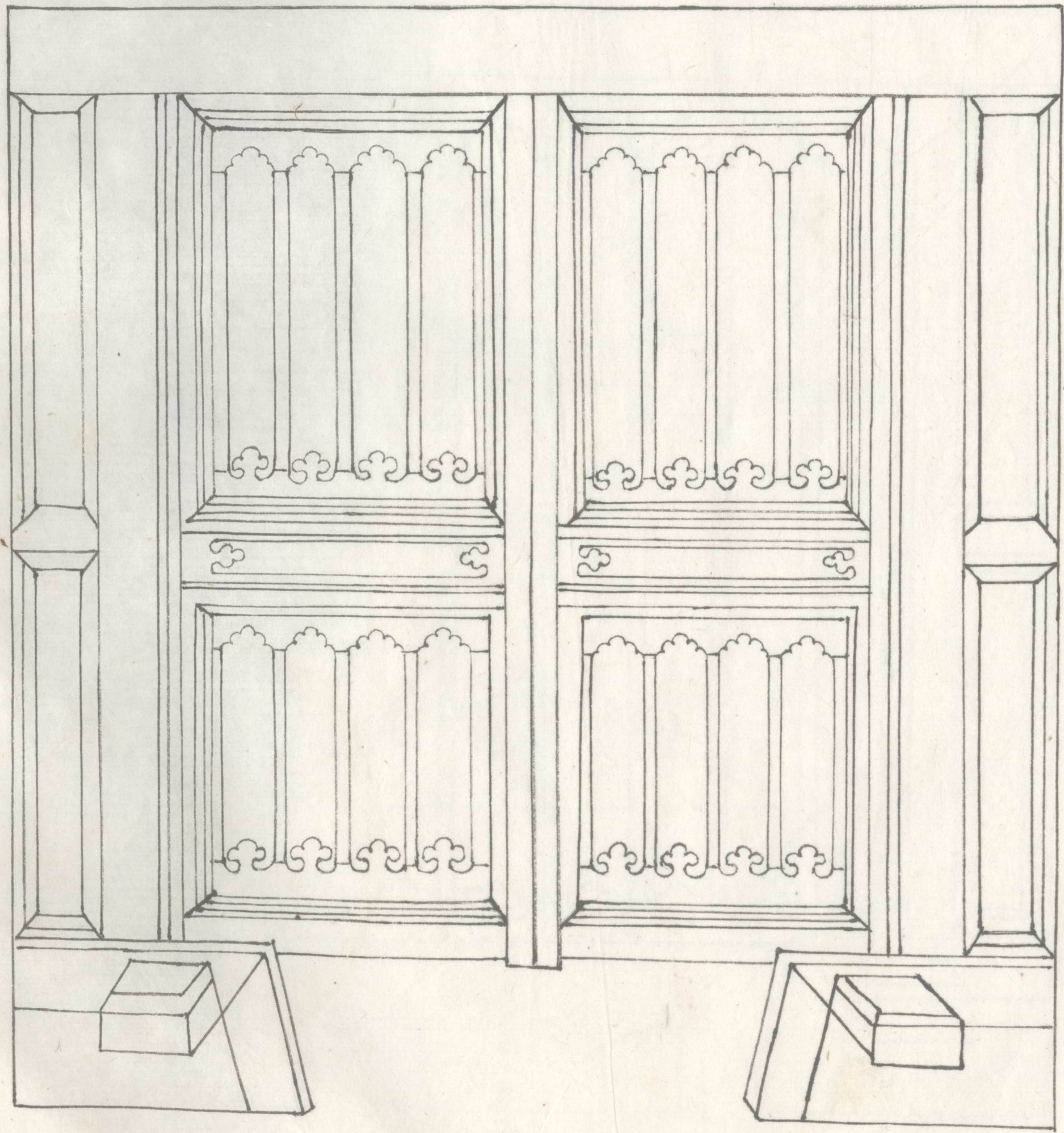
牙頭護縫軟門
