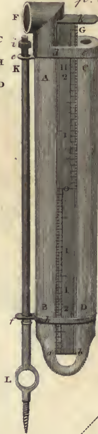
Fig. 4. Wind Gage. p. 661.
