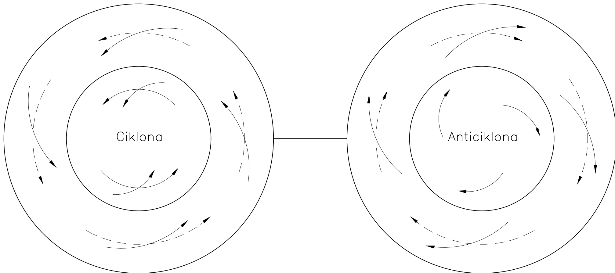
Strujanje zraka pri tlu (—) i u slobodnom sloju atmosfere (---) na sjevernoj polutki: lijevo u cikloni i desno u anticikloni
