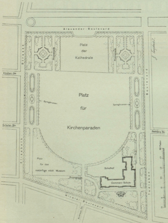
Der neue Plan für die Bebauung und Bepflanzung der Esplanade nach dem Originalentwurf des Stadtgardendirectors S. Kuphaldt. (Vgl. den Artikel „Der Neubau der Rigaer Commerz-Schule“).
