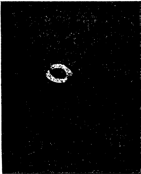
(شكل ٤ - سديم الشلياق الحلقي)
