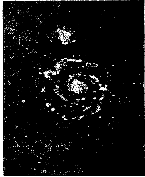
(شكل ١ سديم السلاقي اللولبي)
