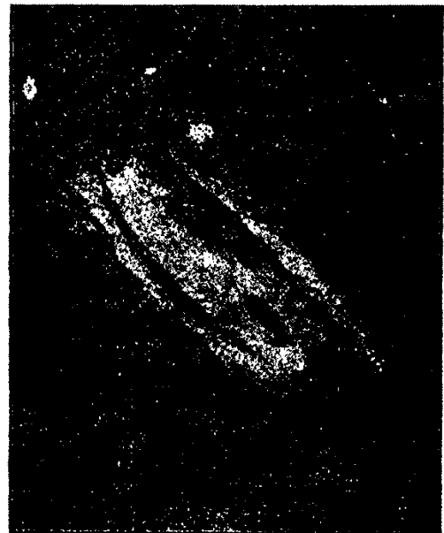
(شكل ٣ سديم المرأة المسلسلة اللولبي)
