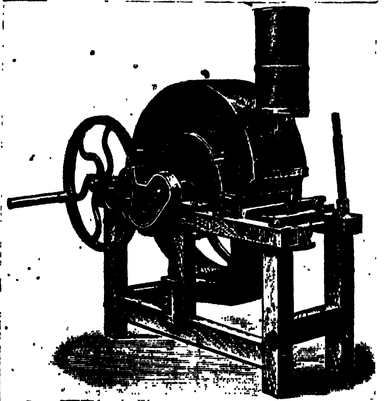
তক্ত-নিক্ষেপনের হস্ত-পরিচালিত কল
