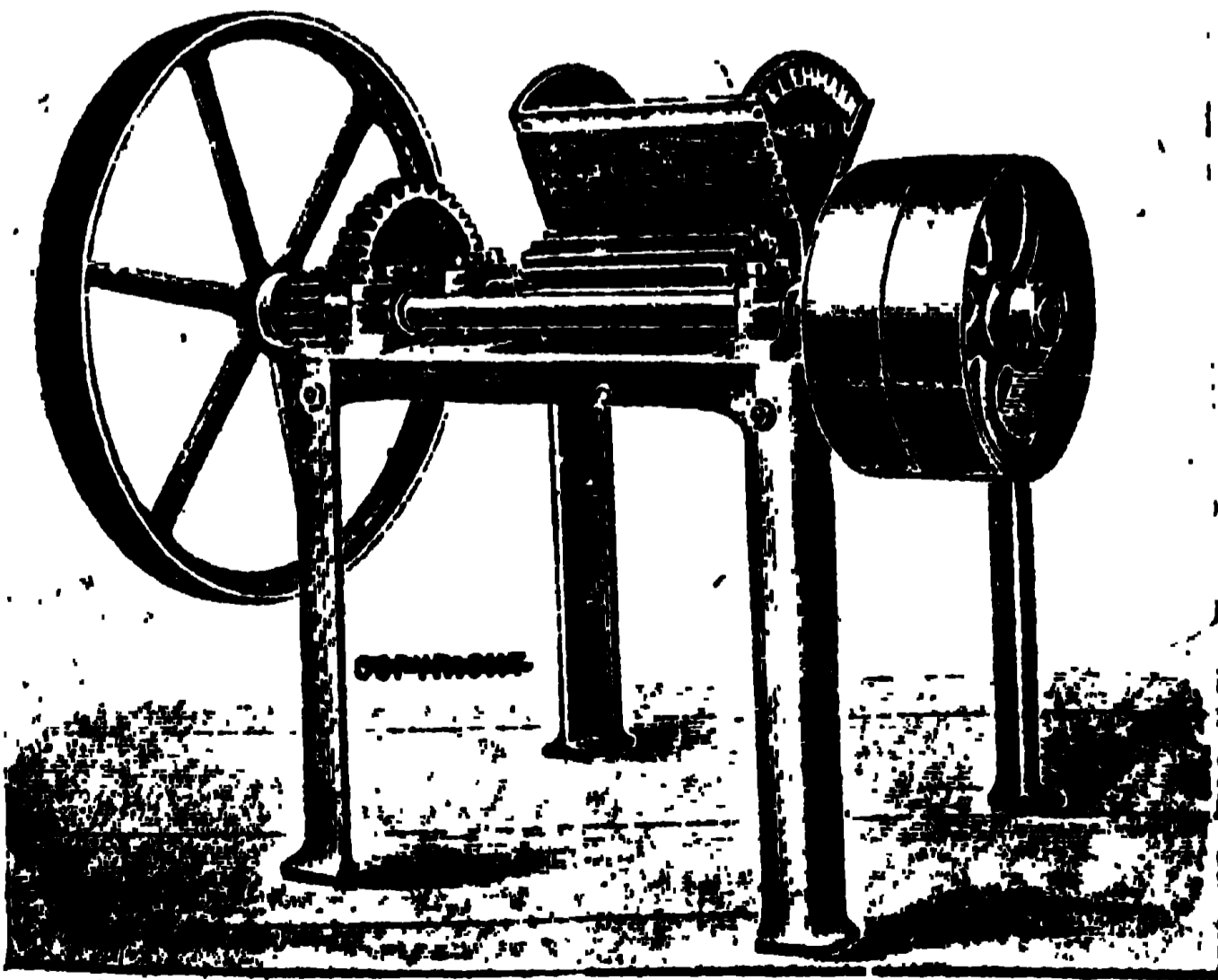
ছোবড়া-পেষণ যন্ত্র
