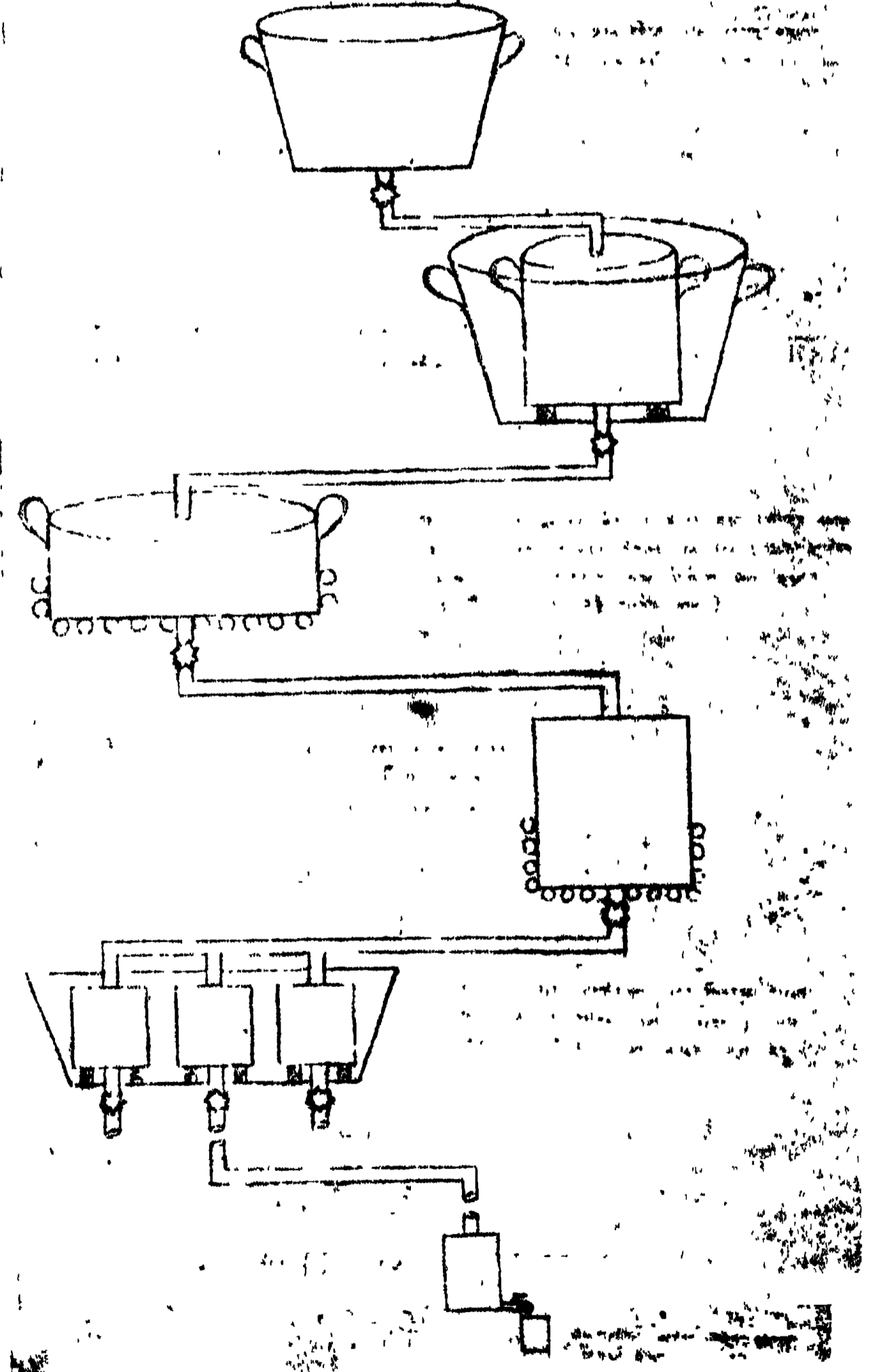
দুগ্ধ গাঢ়-করণ ও সংরক্ষণ প্রকরণ
