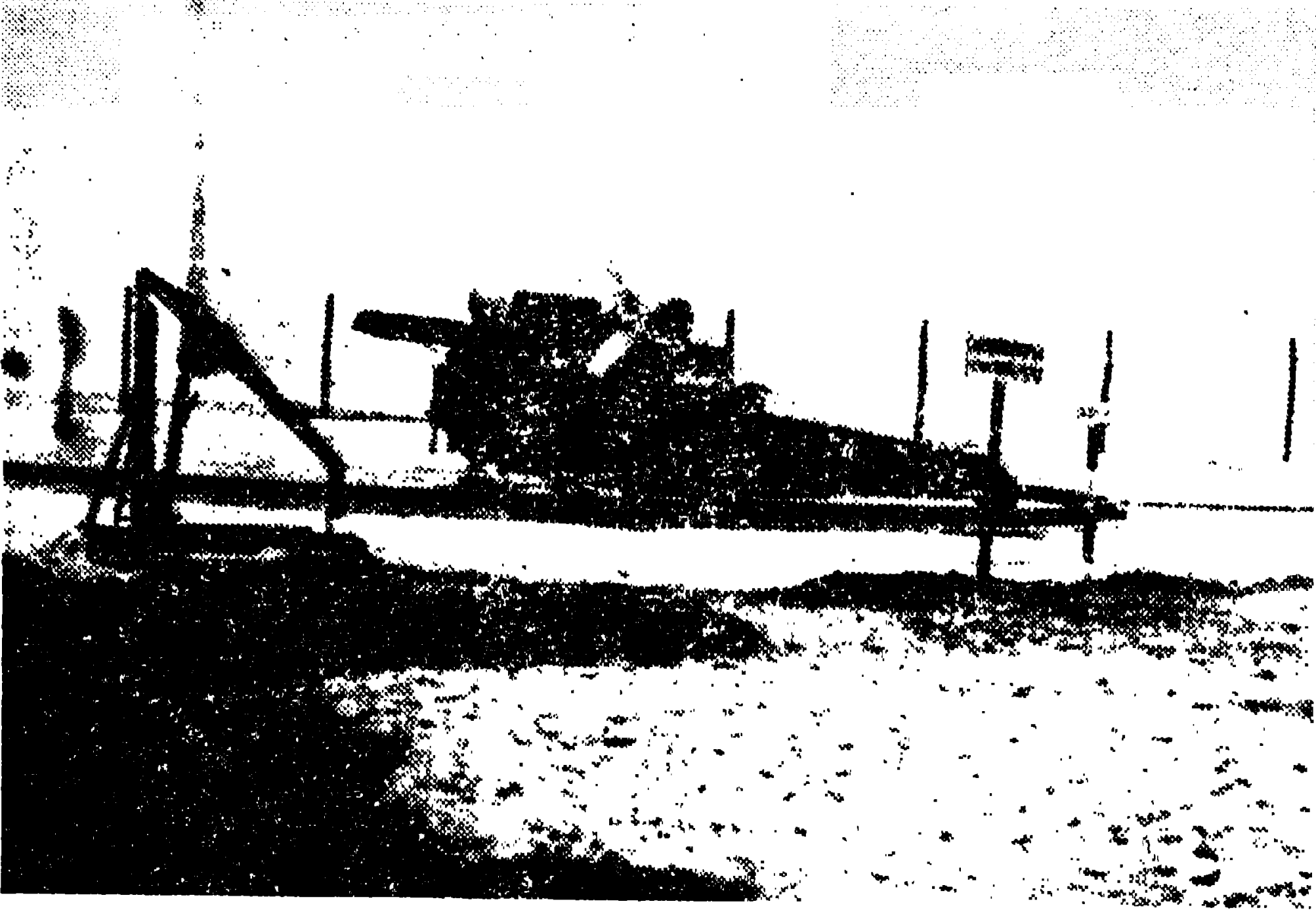
ত্রিবাঙ্গাম থেকে ১৫ মাইল দক্ষিণে যুগ্ম রকেট উৎক্ষেপণ কেন্দ্র
