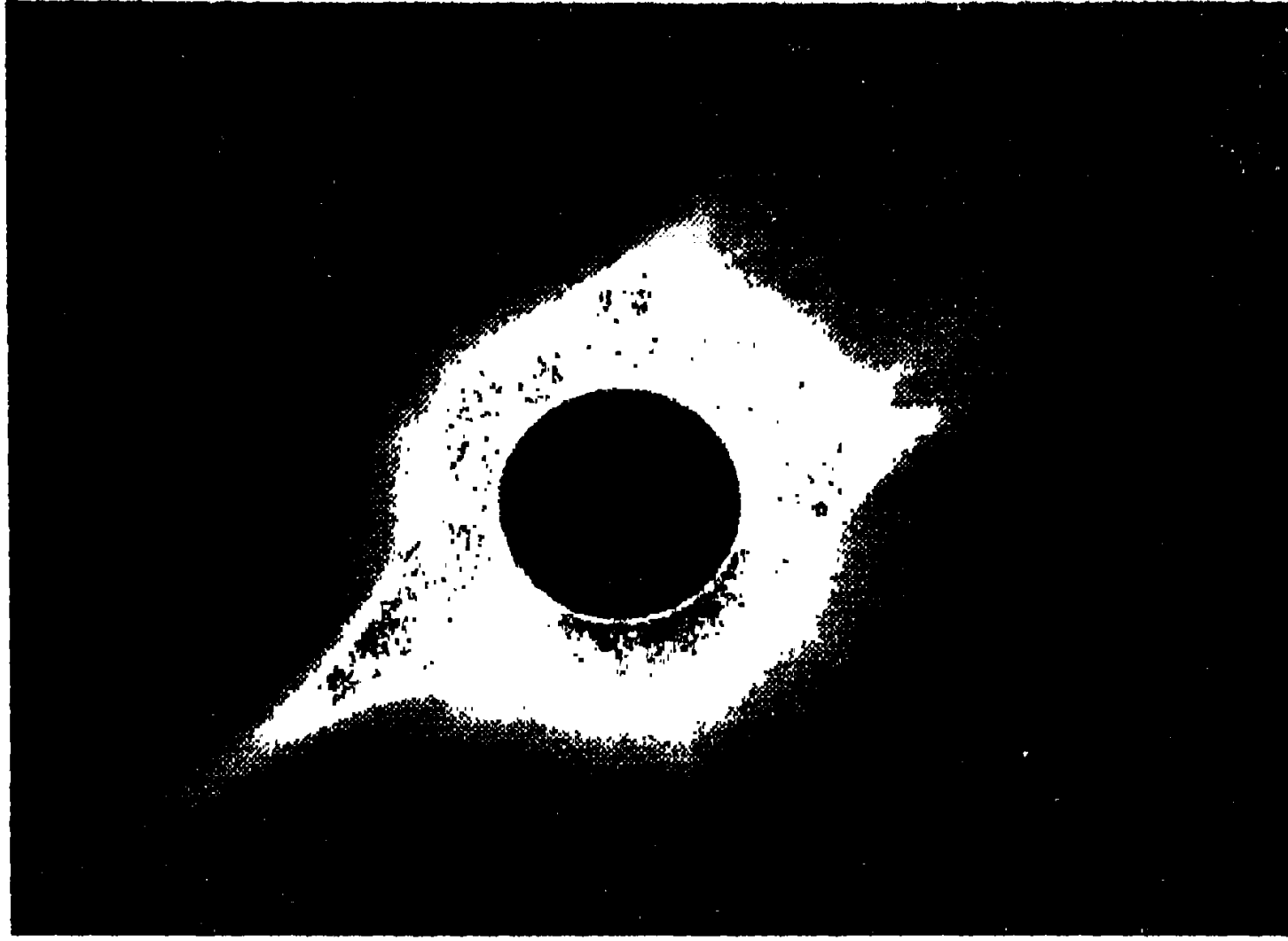
সূর্যকলঙ্ক যখন খুব কম, সেই অবস্থায় পূর্ণ গ্রহণের সময় সূর্যশিখার ছবি
