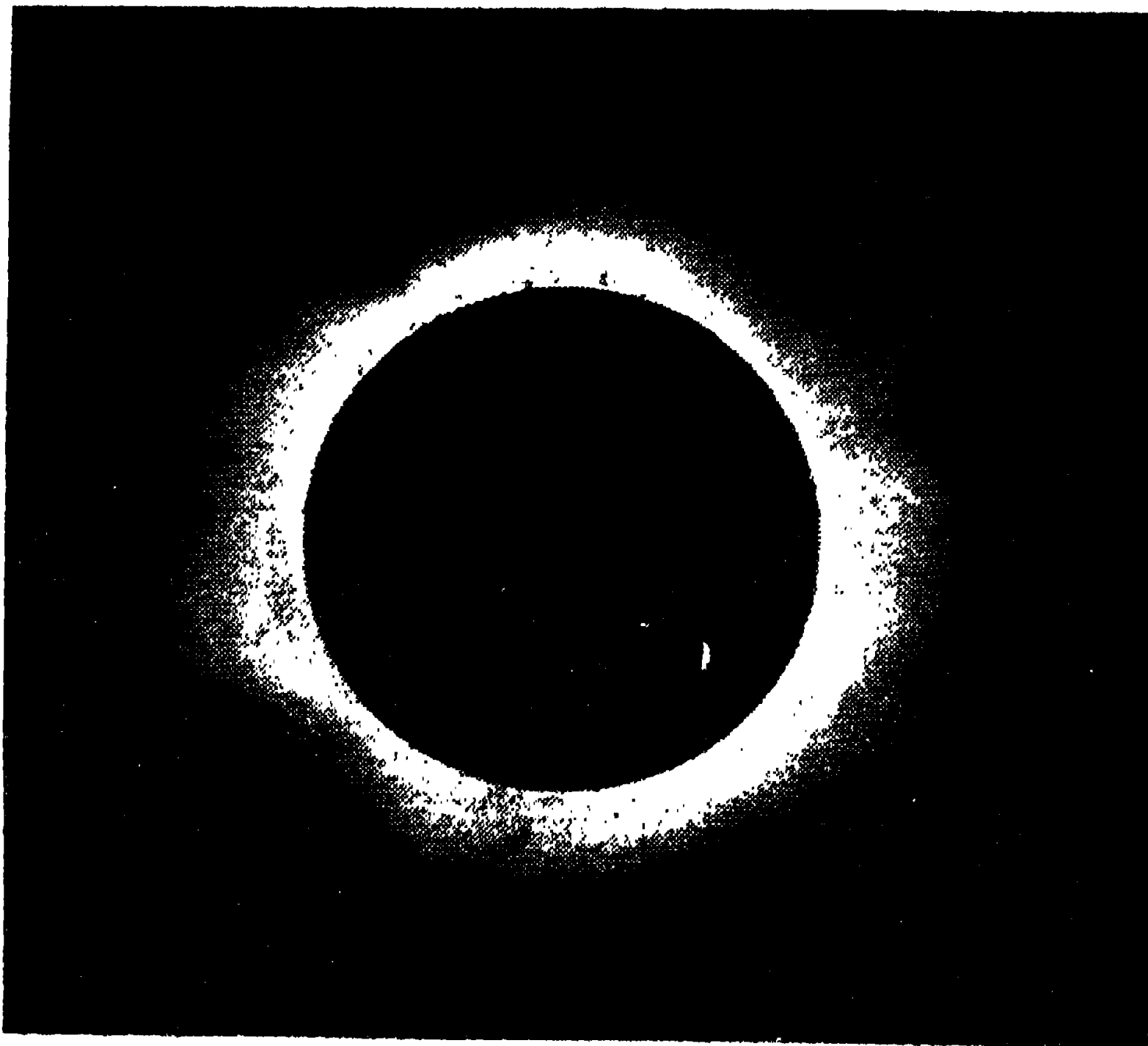
সূর্যে কলঙ্কের প্রাকৃতিক বধন খুব বেশী, পূর্ণ গ্রহণে সেই সময়কার সূর্যশিখার ছবি
