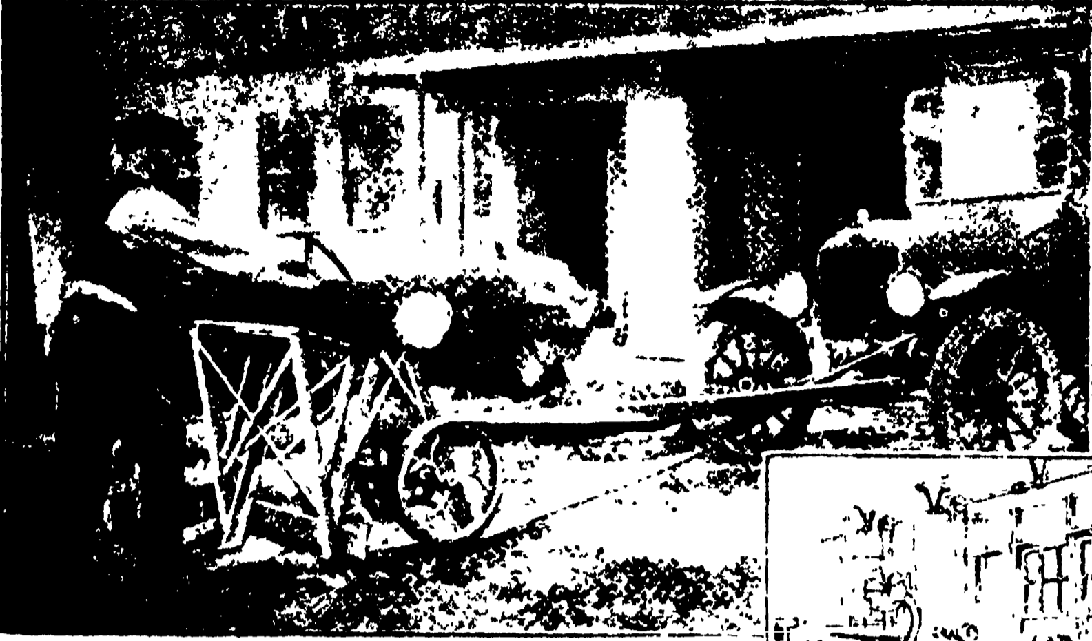
ফোর্ড মোটরের সাহায্যে কেমন ভাবে কাণ্ডানার কাজ চলে দেখুন। বাঁ দিকে কাত কল, ডান দিকে ছোট কারখানা চলিতেছে
