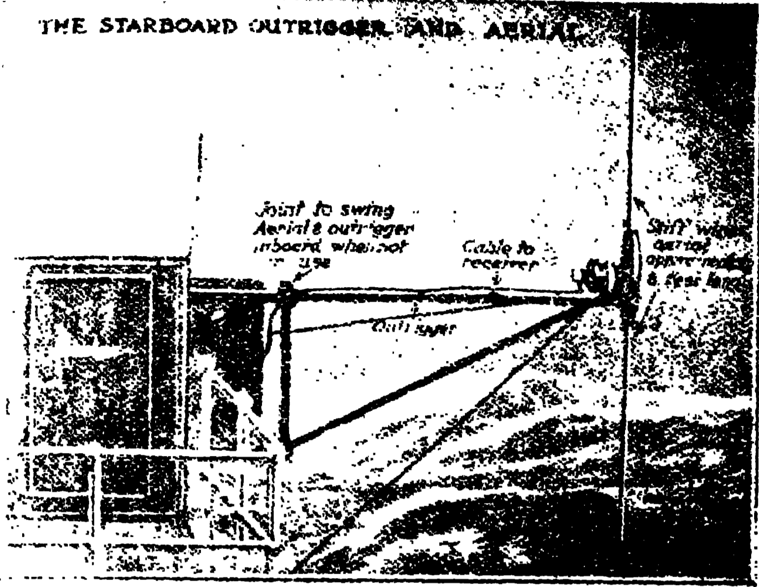
বেতার এরিয়াল (aerial)
