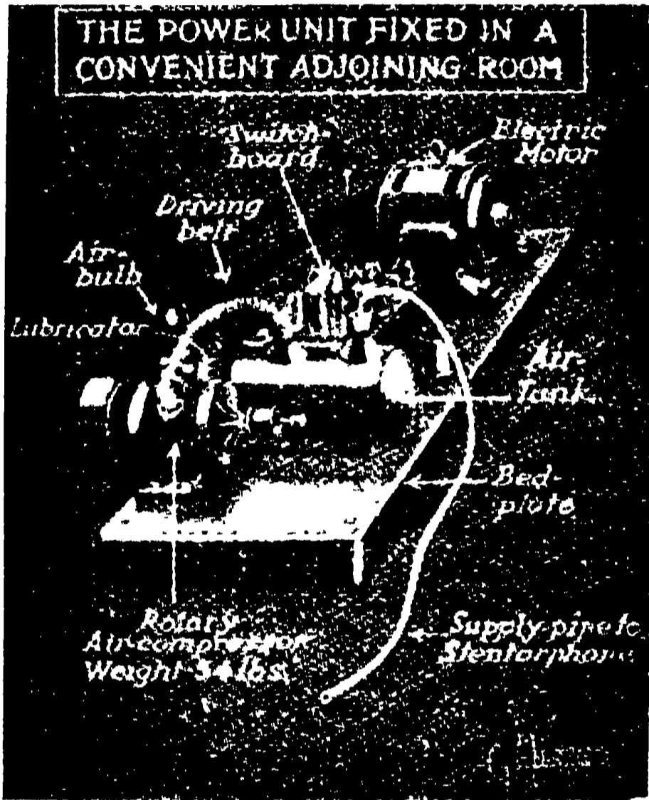
স্টেন্টোফোন চালাবার যন্ত্র (নিকটবর্তী কোনও একটি ঘরে এই যন্ত্র রেখে এর সাহায্যে স্টেন্টোফোন বাজাতে হয়)
