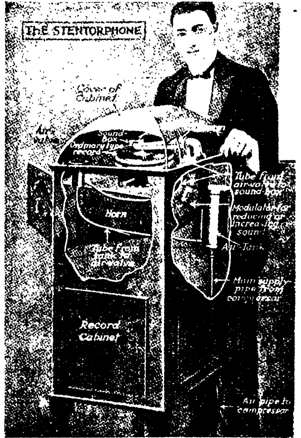
স্টেন্টোফোন
