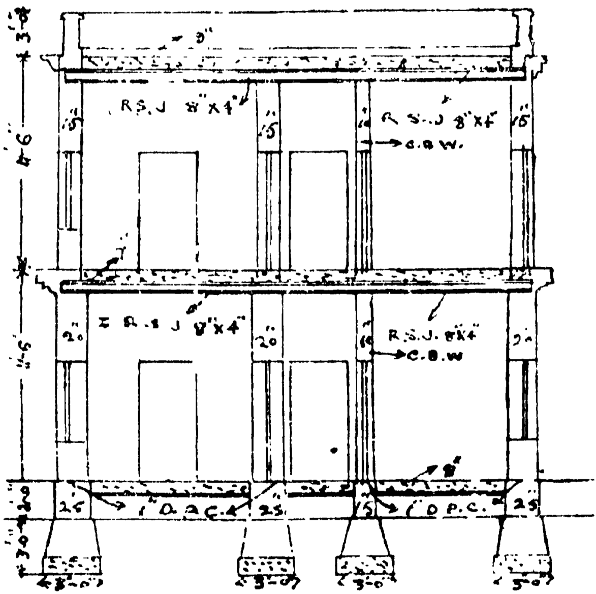
সস্তা বাড়ীর নক্সা
