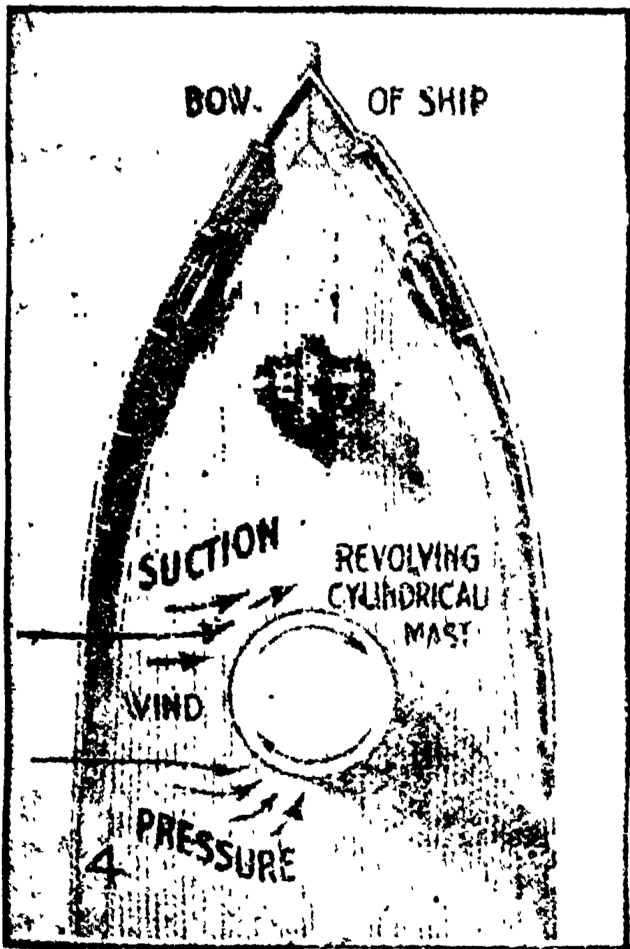
বায়ুর চাপে জাহাজের গতিবৃদ্ধি
