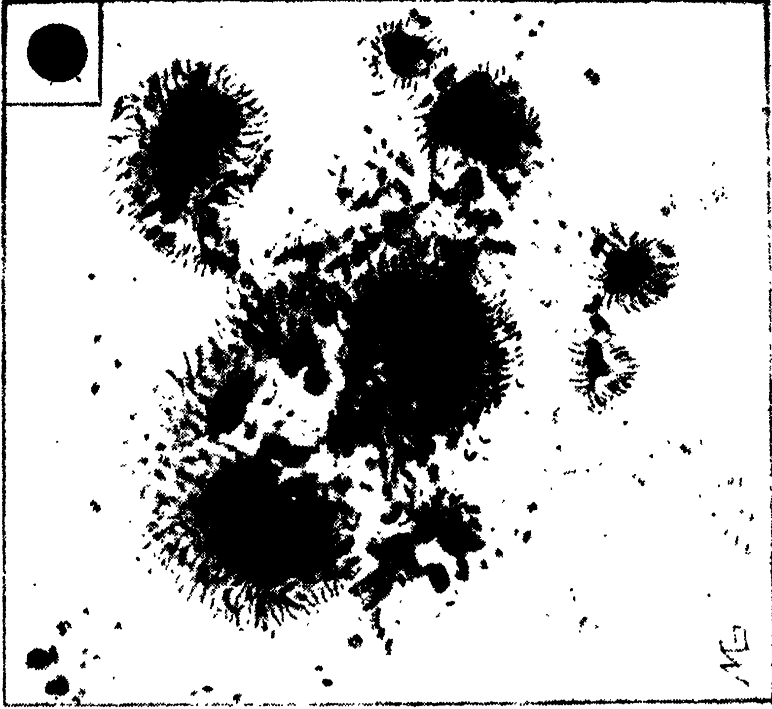
সৌরকলঙ্ক
