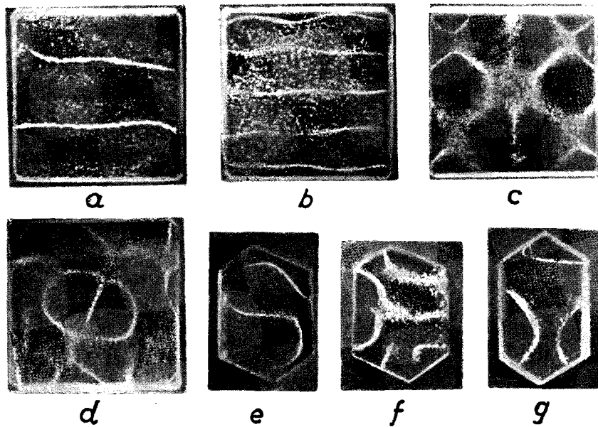
Sl. 4. CHLADNIJEVI LIKOVI NA PLOČICAMA OD KVARCA (pokuši i snimke D. Pejnovića 1935)
