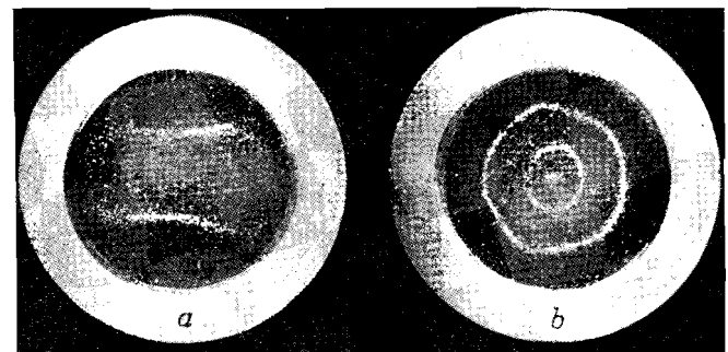
SI. 2. PJEŠĆANE SLIKE NA OKRUGLOJ PLOČI (po D. C. Milleru); frekvencije: 977 (a), 2460 (b)
