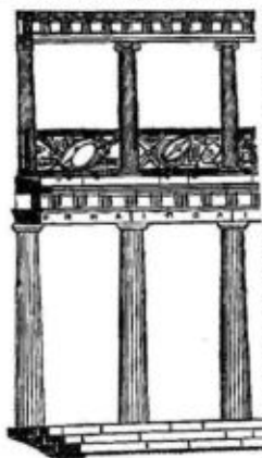
Рис. 1. Двухэтажный портик (стоа) в Пергаме. Реконструкция.
