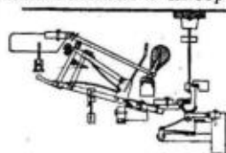
Фортепианная механика Э.
