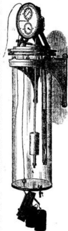
Рис. 3. Нормальные часы № 67.
