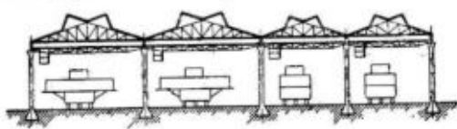
Рис. 4. Эллинги судостроит. завода в Перми.
