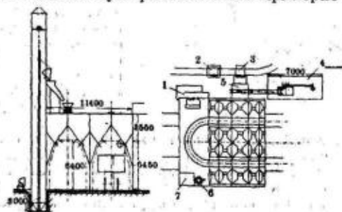
Рис. 8. 1—лестница, 2—весы, 3—кузов вагона, 4—будка подъемного механизма, 5—шахтный подъемник, 6—бак для воды, 7—будка для 3 грузчиков.
