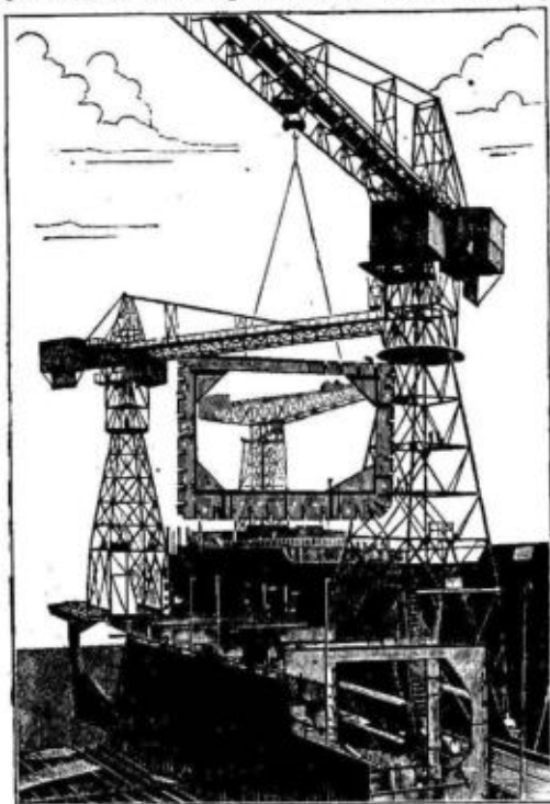
Рис. 2. Эллинг завода Говальд.
