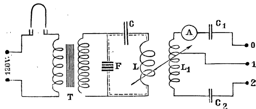
Рис. 1. Схема аппарата для Д.
