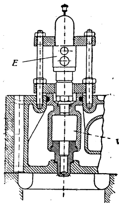
Рис. 5. Предкамера дизеля Кертинг; E —форсунка, V —камера.
