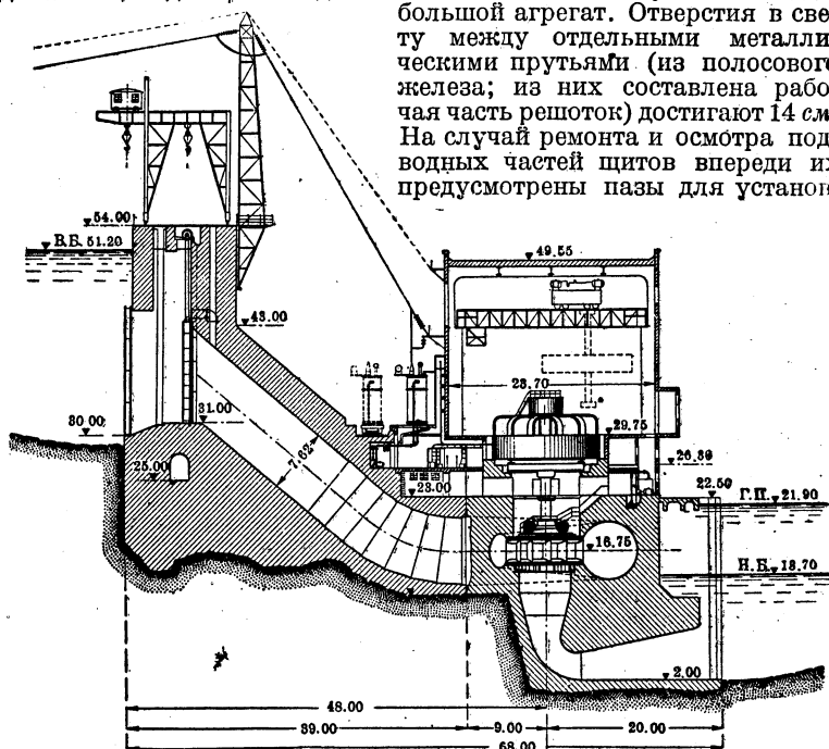
Рис. 4. Поперечный разрез гидростанции.
