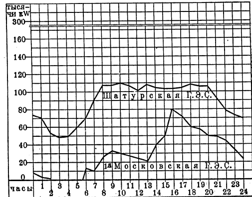
Рис. 3. Суточная нагрузка 1-й МГЭС за 25 апреля 1933 и ШАГЭС за 23 декабря 1933.
