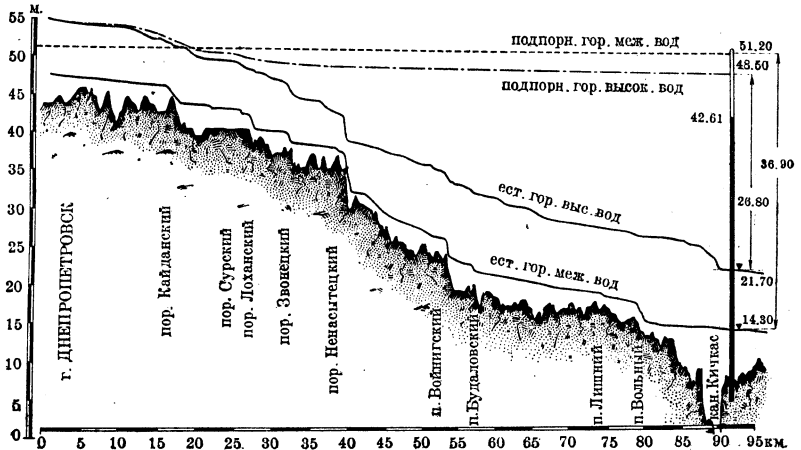
Рис. 1. Продольный профиль порожистого участка р. Днепр.
