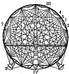
Рис. 3. Схематический разрез пепелина (LZ 127). I—несущий газ-водород; II—газообразное горючее (для моторов); III—шпангоут; IV—киль; 1—внешняя оболочка; 2—одна из 28 сторон главного сечения, образованного сторонами шпангоута и его малой стойкой; 3—боковые моторные гондолы; 4—внутренние стяжки, идущие от каждой стороны; 5—главный стрингер; 6—промежуточные стрингеры; 7—вспомогательный трос; 8—внутренний коридор; 9—пахта для выхода водорода через автоматические клапаны.
