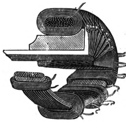
Рис. 9. Устройство якоря.
