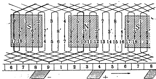
Рис. 11. Обмотка Гейфнер-Альтенека.
