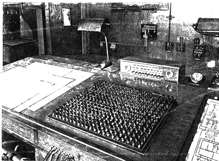
Рис. 6. Стол диспетчера.
