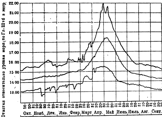
Рис. 2. График колебаний горизонтов Днепра на створе сооружаемой плотины. Кривые показывают горизонт колебаний в маловодный год, максимально многоводный и средний гидрологический.
