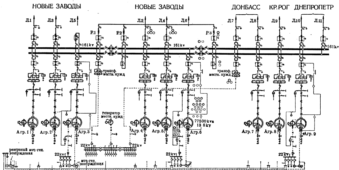
Рис. 7. Однолинейная генеральная схема электрических соединений станции.
