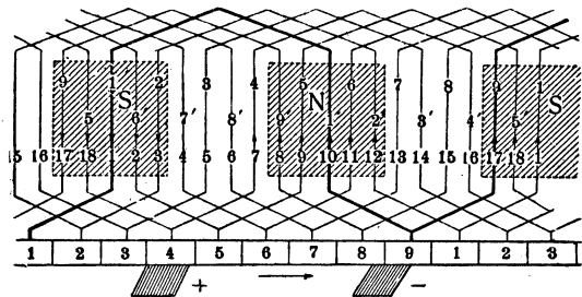
Рис. 12. Волновая обмотка.
