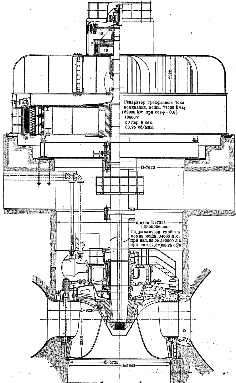
Рис. 6. Продольный разрез по оси главного агрегата.
