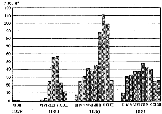
Рис. 5. Суммарный месячный график бетонной кладки по основным сооружениям от начала работ до конца 1931 в тыс. м 3 .
