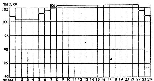
Рис. 4. График напряжений за 14 янв. 1934 на Карачаровской подстанции Мосэнерго.
