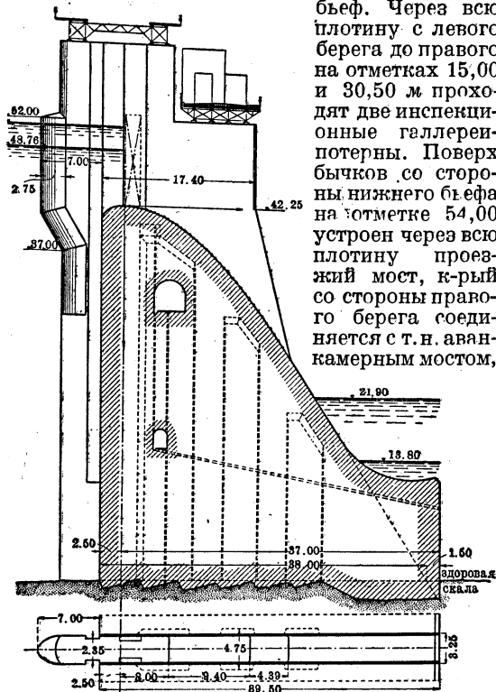
Рис. 2. Нормальный профиль плотины.
