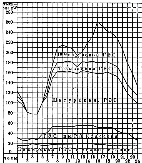
Рис. 2. Суточная нагрузка станций Мосэнерго за 23 декабря 1932.
