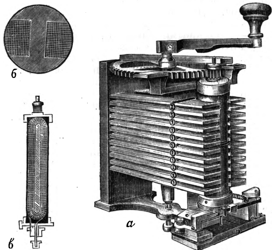
Рис. 5. а—магнито-электрич. машина с якорем Сименса, б—поперечный, в—продольный разрезы якоря.
