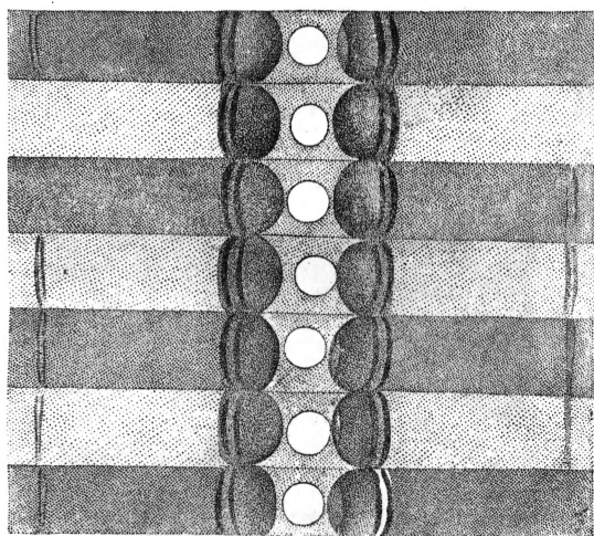
Рис. 8. Смещение линий на рентгенограмме при растяжении диораломина.
