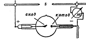
Рис. 3. Схема трубки Кулиджна; s—предохранительный разрядный прожектор.
