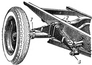
Рис. 1. Задняя Р. автомобиля ГАЗ-АА.
