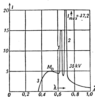
Рис. 2: I —интенсивность Р. л. в относительных единицах; 1 и 2—характеристические линии молибдена (K-серия); 3—сплошной спектр.
