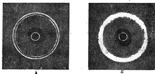
Рис. 9. Холоднотянутая проволока из электролитического железа. Отражение излучения кобальта от плоскости на отожженном (А) и неотожженном (Б) образцах.
