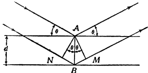
Рис. 2. Разность хода лучей при отражении от двух последовательных плоскостей NB + BM = 2d \sin \theta .
