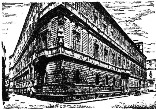
Рис. 10. Палаццо Канцеллария.
