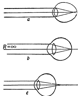
Ход лучей при различной рефракции: а—близорукость, б—эмметропия, с—дальнозоркость.
