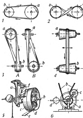
Ременная передача.
