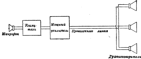
Рис. 2. Схема мощного громкоговорящего телефона по проводам.
