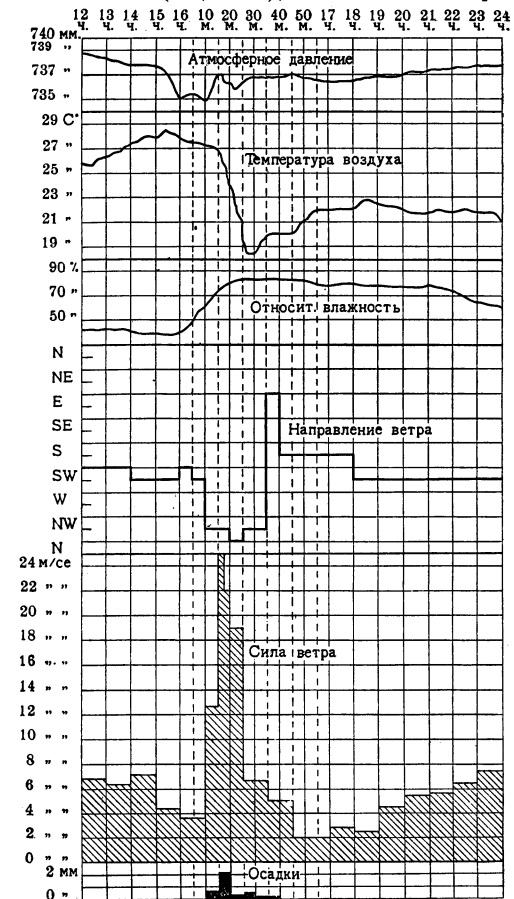
Рис. 1. Записи регистрирующих метеорологических приборов во время грозы.
