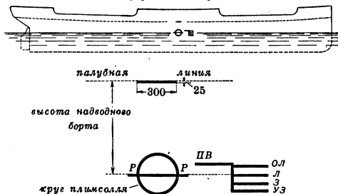
Положение грузовой марки на борту парохода и ее детали. Обозначения: Р-Р—регистр СССР, ПВ—углубление в пресной воде, Л и ОЛ—углубление в соленой воде летом, З и УЗ—углубление в соленой воде зимой.
