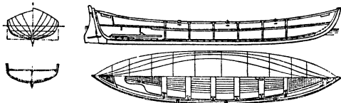
Шестивесельный вельбот.
