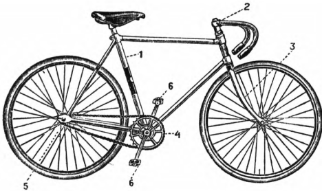
Рис. 1. Тип гоночного велосипеда для трека.
