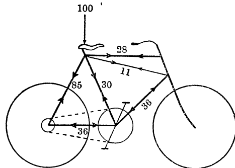
Рис. 4. Схема сил, действующих в раме велосипеда (в кг).
