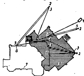
Рис. 5. Схема канатно-тяговых установок при передвижении по криволинейному пути: 1—лебедка; 2—мертвяк; 3—четыре блока; 4—один блок; 5—два блока; 6—прикрепление к дому; 7—контур начального положения дома; 8—контур дома после поворота.
