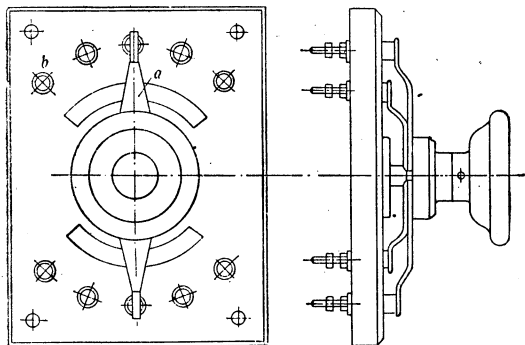
Вольтметровый переключатель: а—вращающаяся часть П.; б—неподвижные контакты.
