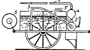
Рис. 2. Разрез пеногона типа «Тремасс».
