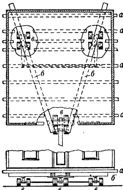
Рис. 1. Опорная рама для легких зданий: а—поперечные балки; б—продольные балки; в—тепелки.
