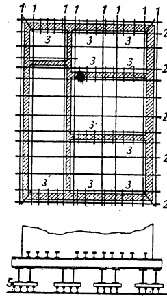
Рис. 2. Опорная рама для зданий среднего и крупного веса: 1—ходовые балки; 2—поперечные балки; 3—короуши; 4—катки; 5—рельсы.
