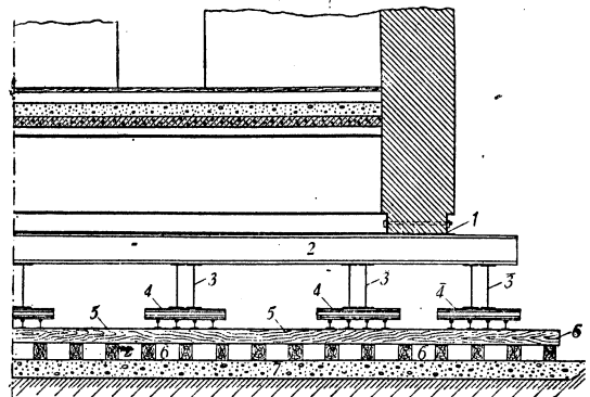
Рис. 3. Деталь расположения элементов опорной рамы: 1—обвязочные балки; 2—поперечные балки; 3—ходовые балки; 4—катки; 5—рельсы; 6—брусья основания; 7—бетонная подготовка.
