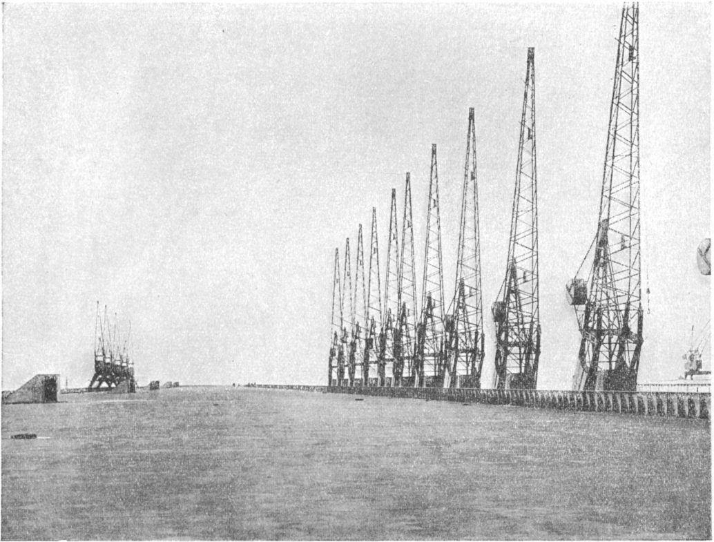
Л и в е р п у л ь. Подъемные краны нового дока (так называемый док Гладстона, 460 м длины).
