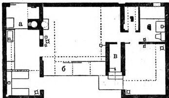
Рис. 3. Американский одноэтажный бетонный дом. Рассчитан на массовое строительство. Наверху дома спальные террасы. Предназначается для юж. климата (Флорида).
