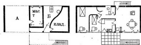
Рис. 4. Тип современного дома-особняка по идее Корбюзье. Дом одноэтажный на столбах. На крыше сад с крытой террасой. Буквы А и Б обозначают открытые дворы.
