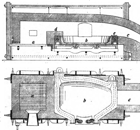
Рис. 3. Пудлинговая печь.
