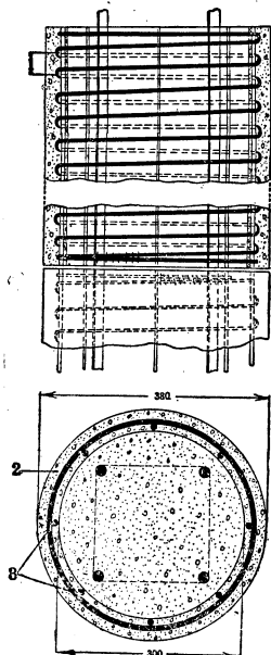
Рис. 11. 1—шаг 50, 2—бетонный стакан со спиральной арматурой, 3—вертикальные прутки.
