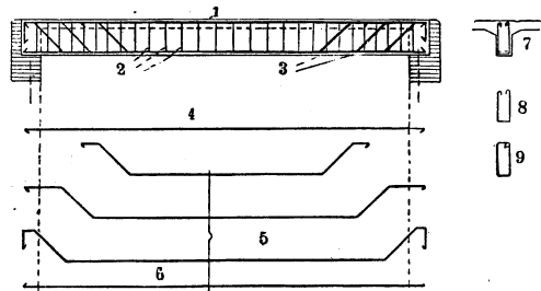
Рис. 4. 1 — монтажное железо, 2 — хомуты, 3 — рабочая арматура, 4 — два монтажных стержня, 5 — рабочие стержни, 6 — прямые стержни (не менее двух), 7 — поперечное сечение, 8, 9 — формы хомутов (8 — открытая, 9 — замкнутая).
