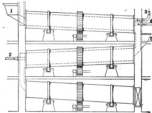
Рис. 2. 1—руда, 2—горелка, 3—дутье, 4—пыль, 5—уголь для восстановления.
