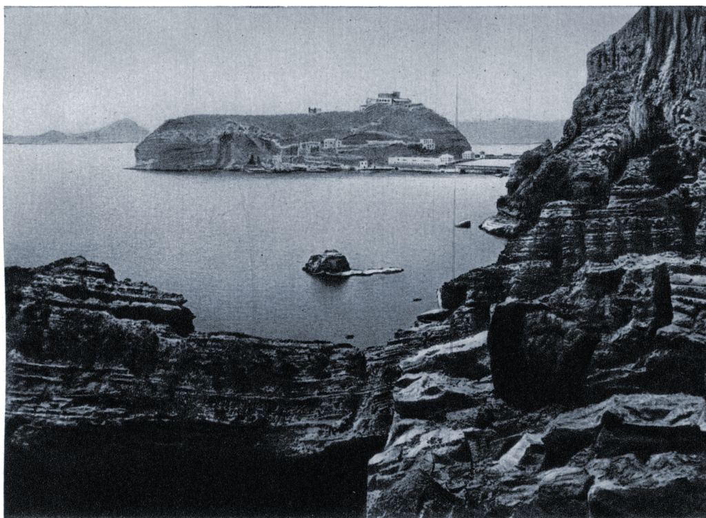
Вулканический островок Низида близ Неаполя (на первом плане скалы из вулканических туфов у Позилипо).
