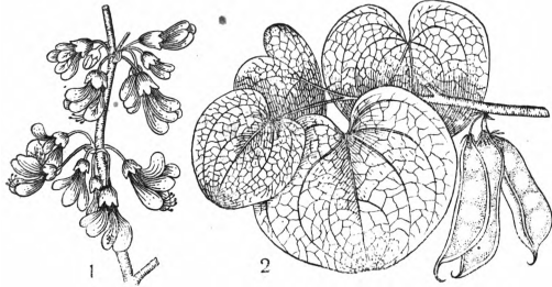
Cercis siliquastrum : 1—ветка с цветами, 2—ветка с плодами.
