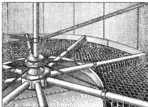
Рис. 3. Поддача воды в охладители Сегнеровым колесом.
