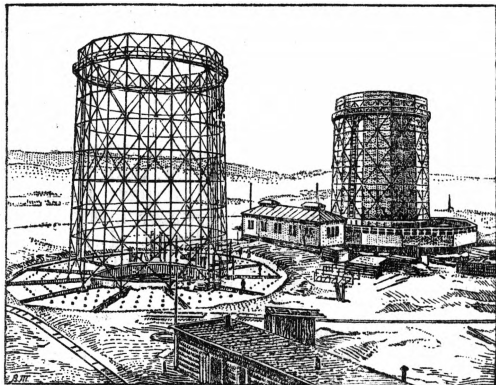
Рис. 2. Башенный охладитель.
