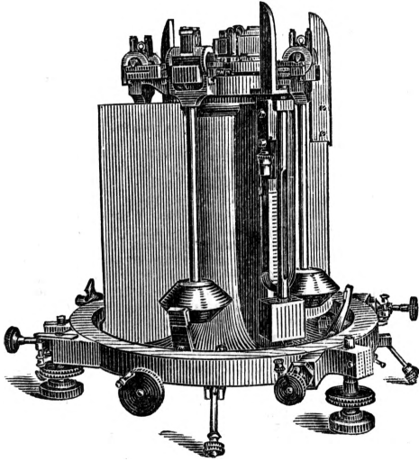
Рис. 3. Маятниковый аппарат Штюкрата-Штернса.
