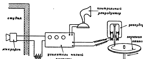
Рис. 2. Схема электромагнитной граммофонной записи.
