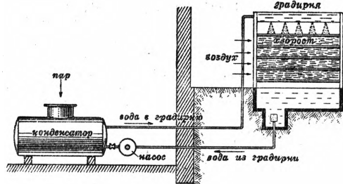
Рис. 1. Схема установки градирни.
