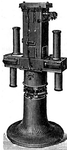
Рис. 5. Крутильные весы (гравитационный вариометр) системы Швейдара.
