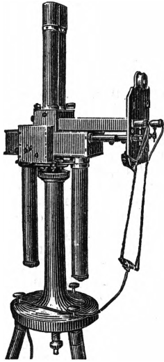
Рис. 6. Крутильные весы (гравитационный вариометр) системы СОФМИ—ИИП.
