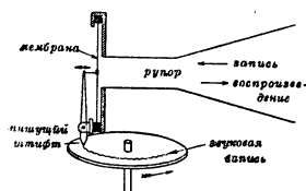
Рис. 1. Схема акустической записи и воспроизведения.
