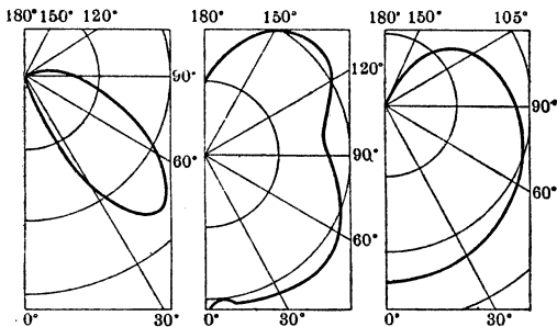
Рис. 5. Г. распределения света для трех разных типов дуговых фонарей.
