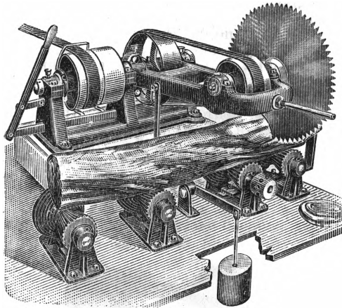
Рис. 4. Балансирующая пила.
