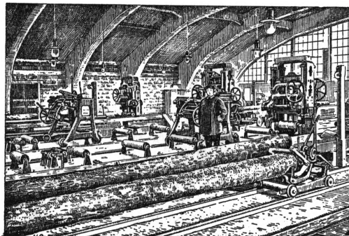
Рис. 2. Рамный цех нового механизированного Дубровского лесопильного завода Севзаплеса.
