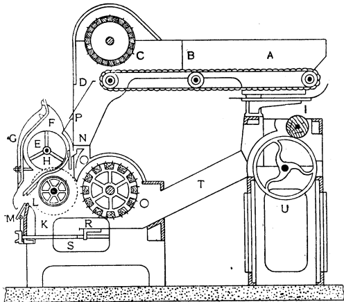
Рис. 2. Пильный джин.
