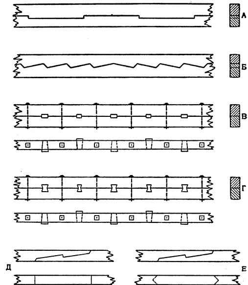
Рис. 1. А—замок накладными прямыми зубьями, Б—замок накладными косыми зубьями, В—замок с косцами, Г—замок с двойным свордовником, Д—замок с косозубом, Е—замок с резкой на ус.
