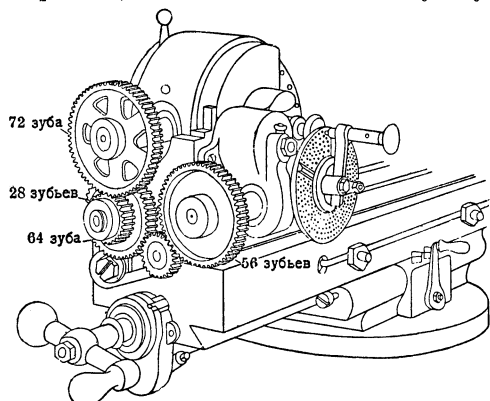
Рис. 2. Дифференциальное деление при помощи двойной зубчатки.
