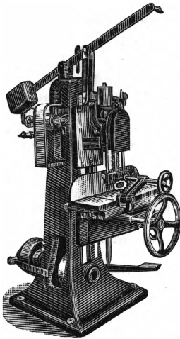
Рис. 8. Долбежный станок.
