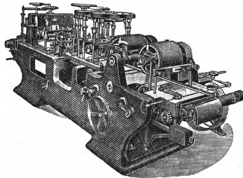
Рис. 6. Строгальный станок с 5 ножами.
