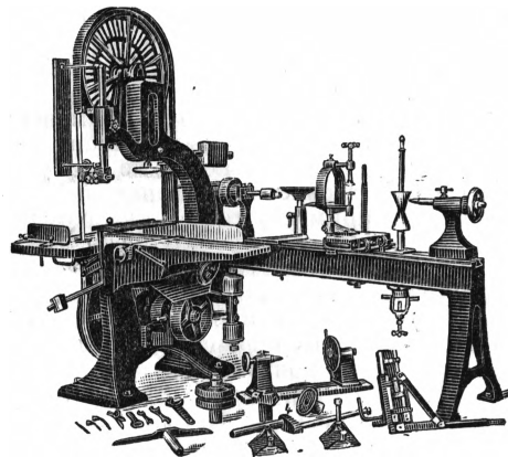
Рис. 10. Комбинированный деревообделочный станок.
