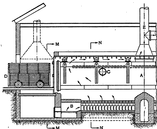
Рис. 6. Установка из 2 американских стандартных реторт.
