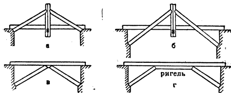
Рис. 6. а—г—подвесные и подкосные системы для перекрытия пролетов мостов.
