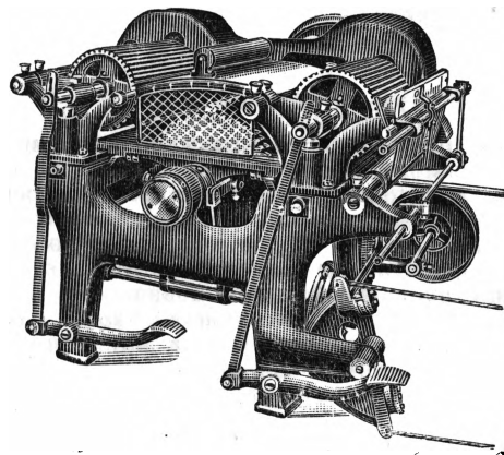
Рис. 3. Обрезной станок.
