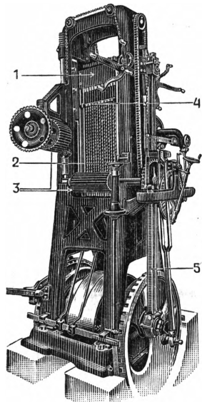
Рис. 1. Лесопильная рама немецкого типа (двухшатуновая): 1 — рама, 2 — пильные полотна, 3 — ролики для бревен (верхний открыт), 4 — прокладки между пилами, 5 — шатуны.
