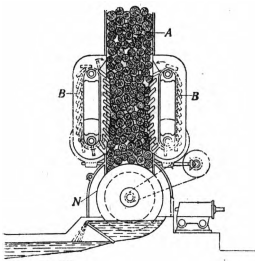
Рис. 2. Схема устройства непрерывного дефибрера Фойта.
