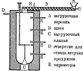
Рис. 7. Реторта Стаффорда.
