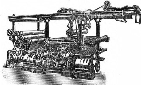
Рис. 2. Мокрый декатир.
