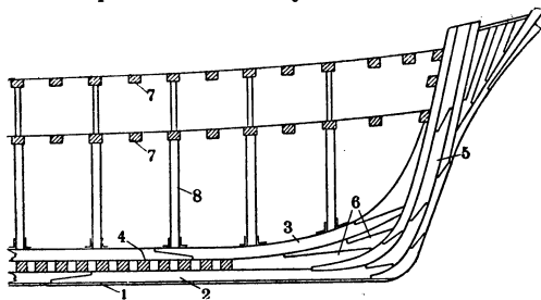
Рис. 3. 1—киль, 2—фальшкиль, 3—кильсон, 4—флортимбер, 5—стем, 6—дедвуд, 7—бимсы, 8—пиллерсы.
