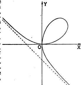
Декартов лист.
