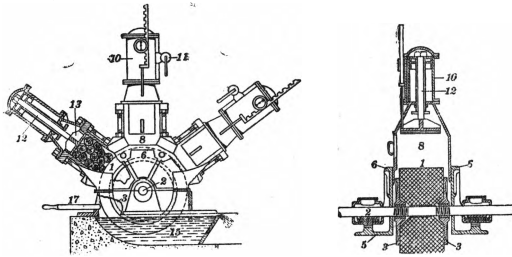
Рис. 1. Гидравлический трехпрессный дефибрер.
