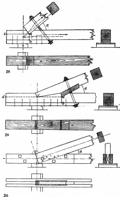
Табл. Д. Основные схемы решения опорного узла деревянных стропильных ферм. Рис. 28. Простая лобовая врубка (зуб). Применяется только в брусовых и бревенчатых решениях. Плохое использование затяжки и подкоса (особенно если последний одновременно не работает на поперечный изгиб от междуузловых нагрузок). При правильной центровке (по сечению a-b ) решающее значение имеет сопротивление складыванию (по a-c ).—Рис. 29. Двойная лобовая врубка (с дубовым вкладышем) при малых углах дает значительно более мощное сопротивление складыванию (по a-c-d ), чем простая врубка.—Рис. 30. Щелевая врубка. Простейшее решение опорного узла досчатых стропильных конструкций. Значительное увеличение ширины и количества скальваемых поверхностей. Простая и ясная центровка.
