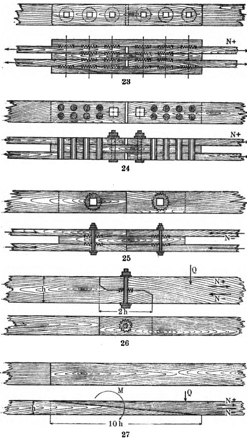
Табл. Г. Рис. 23. Растянутый стык на кольцевых шпонках. Зубчатая кольцевая шпонка при шир. доски в 10 мм.—Рис. 24. Растянутый стык на нагелях. Дубовые нагеля в Д. к., подверженных действию кислотных испарений или паровозного дыма.—Рис. 25. Сжатый стык как правило решается простым лобовым упором. Во избежание продольного изгиба в панели строительной фермы стык располагается около узла и скрепляется болтами и шпонками или гвоздями, рассчитанными по сдвигающим усилиям.—Рис. 26. Стык при наличии одновременно и поперечной силы Q и продольных усилий N+ или N- .—Рис. 27. Универсальный жесткий стык на клею, воспринимающий поперечные и продольные усилия и изгибающий момент—как монолитный брус.
