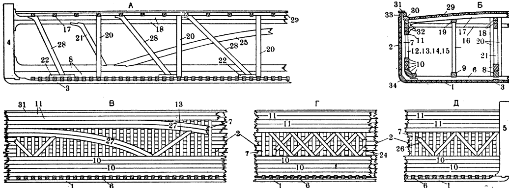
Рис. 7. 1—днище, 2—наружная бортовая обшивка, 3—лыжная, 4—носовой штевень, 5—кормовой штевень, 6—копаны, 7—приставка, 8—средний кильсон, 9—боковой кильсон (третной), 10—воротовые, 11—подбалочные, 12—бортовое внутреннее арочное крепление, 13—раскосы при арках, 14—бортовое внутреннее раскосное крепление, 15—бортовое внутреннее крестообразное крепление, 16—оазы, 17—бимсы, 18—средний конь, 19—боковой конь, 20—схваты, 21—коронные стойки, 22—полунки, 23—шилдерсы, 24—кресты, 25—уголы, 26—раскосы, 27—арочная ферма, 28—коронные раскосы, 29—палуба, 30—ватервейс, 31—плаширь, 32—днища, 33—красная доска, 34—череповой.
