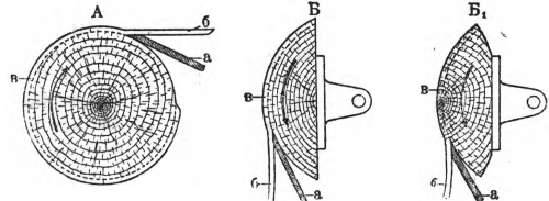
Рис. 5. Схема лущения дерева: А—целого дерева, Б—в полдерева по образующей, Б 1 —в полдерева перпендикулярно образующей, а—лущильный нож, б—снимаемый слой фанеры, в—линия реза.
