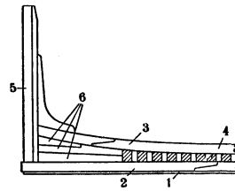
Рис. 4. 1—киль, 2—фальш-киль, 3—кильсон, 4—флор-тимбер, 5—старпост, 6—дедвуд.
