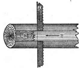
Рис. 4. Схема продольного резания дерева пилой: А—пила и направление ее движения в момент резания, В—бревно и направление его движения на пилу, В—поверхность среза.
