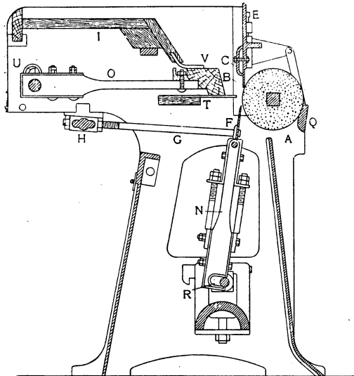
Рис. 1. Валичный джин.
