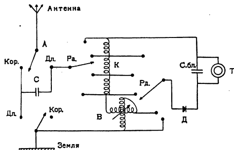
Рис. 2. Детекторный приемник с перемен. дет. связью т. П—8. К—катушка для грубой настройки антенны рычагом Па. Рд.—рычаг для регулирования детекторной связи. В—вариметр для точной настройки антенны. Остальные обозначения те же, что на рис. 1. Диапазон волн 300—1.875 м. Прием длинных и коротких волн так же, как и для приемника т. ПД.
