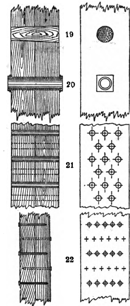
Табл. В. Рис. 19. Дубовый нагель.—Рис. 20. Железный трубчатый нагель.—Рис. 21. Стальные штифты.—Рис. 22. Гвозди (диаметром не более 6 мм).
