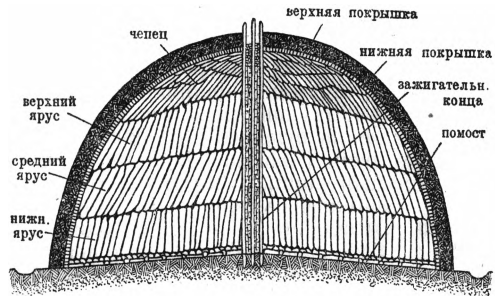
Рис. 2. Стоячая куча для переугливания дерева.
