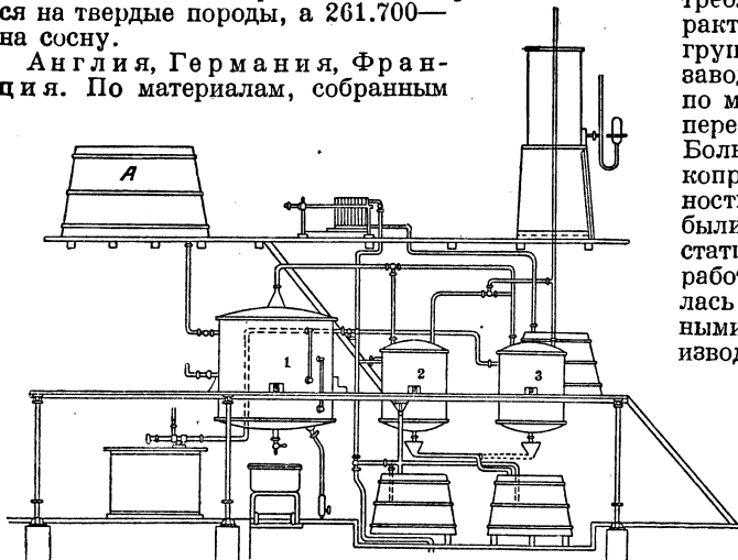
Рис. 8. Трехкубовый аппарат для переработки древесного уксуса.
