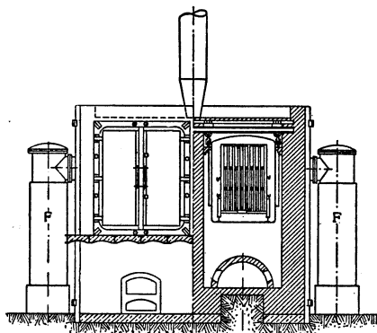
Рис. 6. Установка из 2 американских стандартных реторт.
