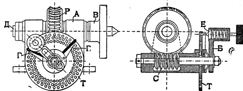
Рис. 1. Делительный аппарат с делительным кружком.
