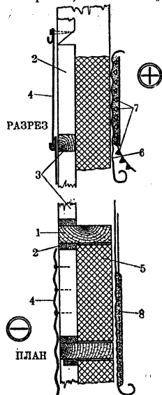
Рис. 4. 1—стойка, 2—прибойна, 3—горизонтальная рейка для укрепления асбестфанеры, 4—волнистая асбестфанера, 5—плиточный утеплитель, 6—изоляция, 7—деревянно-речный мат, 8—штукатурка.
