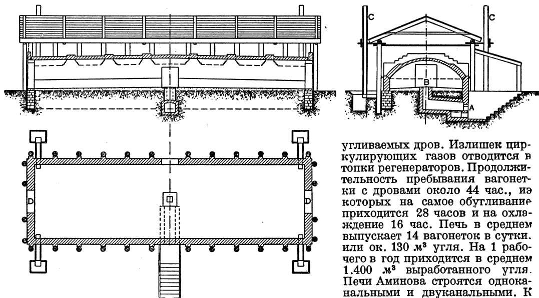
Рис. 3. Печь Шварца уральского типа на 100 м 3 .
