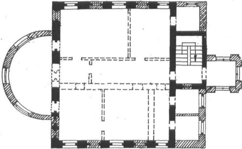
План 2 этажа
