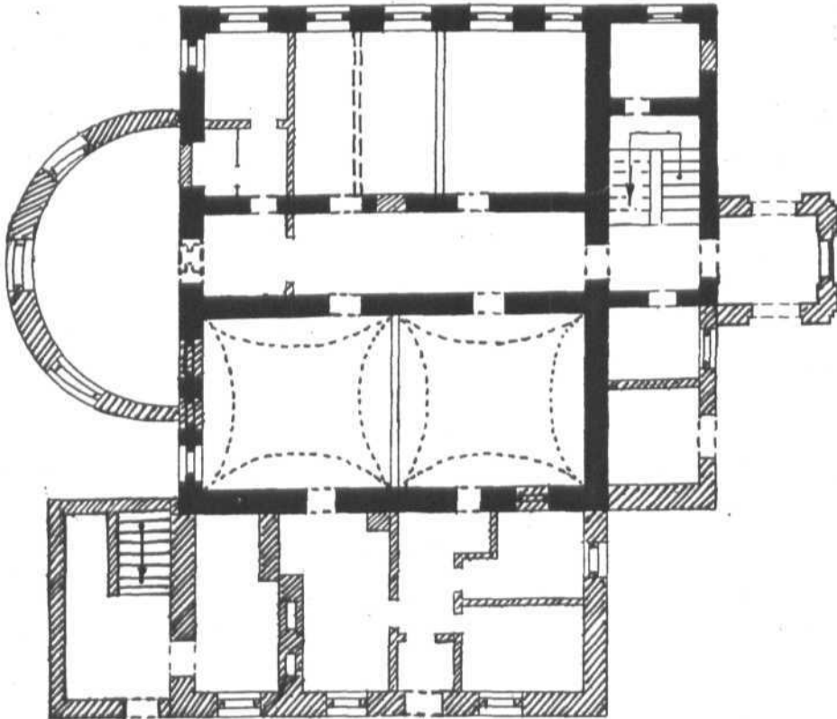
План 1 этажа
